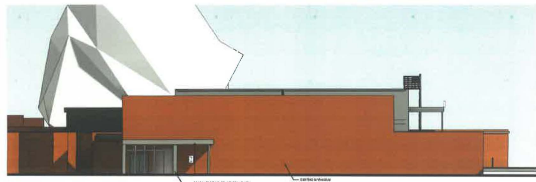
3 NEW GYM VESTIBULE ELEVATION A01 SCALE: 1/8" = 1'-0"
